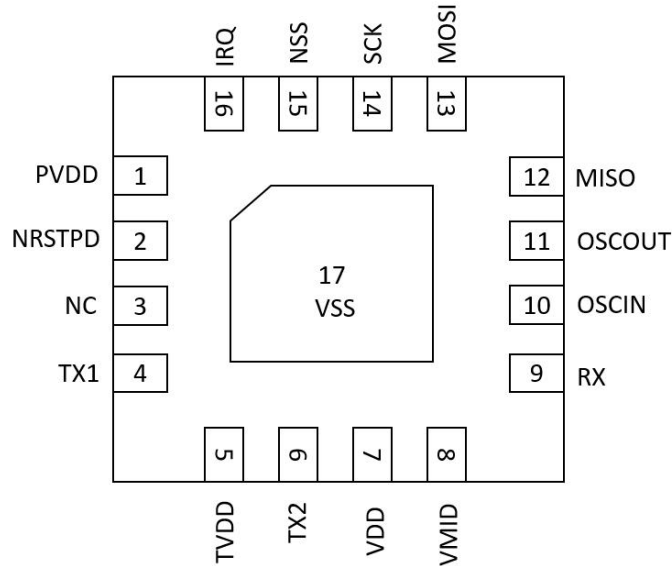
图 1 QFN16 封装脚位图
