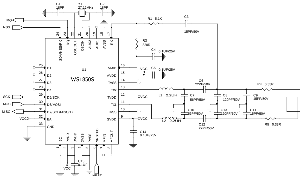
图3 WS1850S双天线应用电路图
