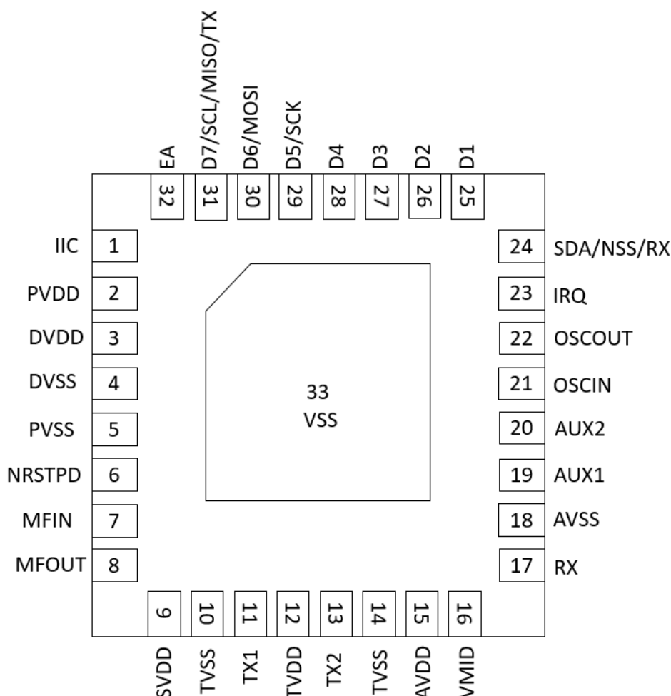
图1 QFN32封装脚位图
