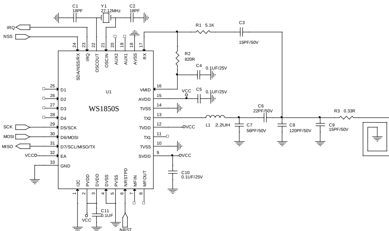
图4 WS1850S单天线应用电路图
